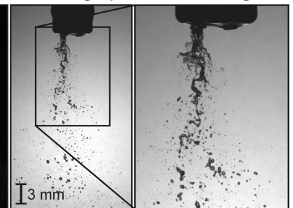
Endoskopische Düse
